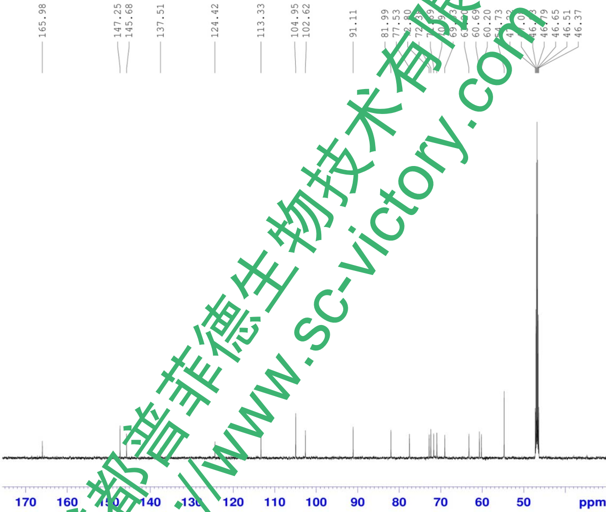
13 C-NMR 图
