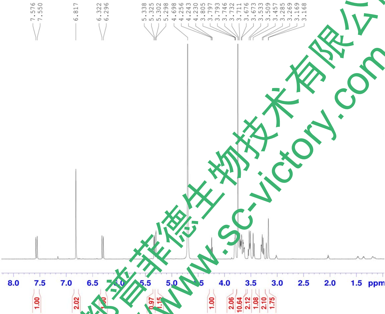
1 H-NMR 图
